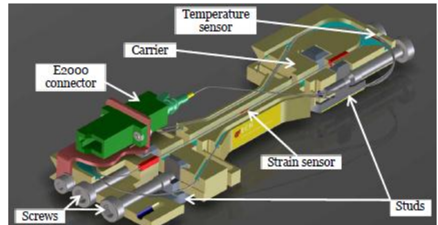
▲ Fig. 1. FOBM sensor
